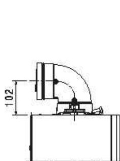
KOAKSIJALNI DIMOVOD Ø60-100 mm
