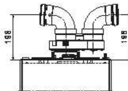
ODVOJENI SISTEM Ø80-80 mm SA ADAPTEROM
