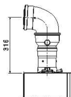
KOAKSIJALNI DIMOVOD Ø80-125 mm
