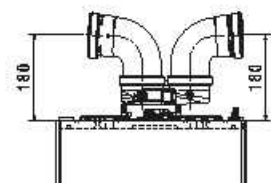
ODVOJENI SISTEM Ø80-80 mm SA KOMPAKTNIM ADAPTEROM
